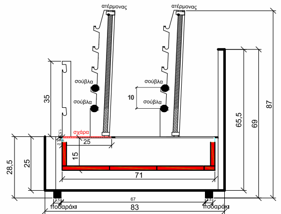
ΠΛΑΪΝΗ ΟΨΗ 2 ΑΞΙΟΝΑΣ
