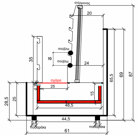
ΠΛΑΪΝΗ ΟΨΗ 1 ΑΞΙΟΝΑΣ
