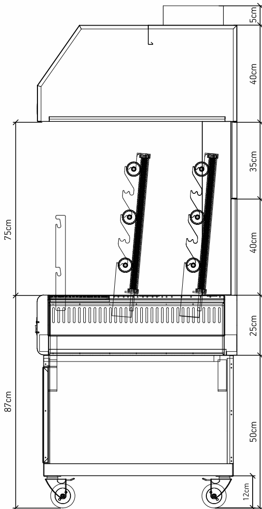
ΠΛΑΪΝΗ ΟΨΗ
