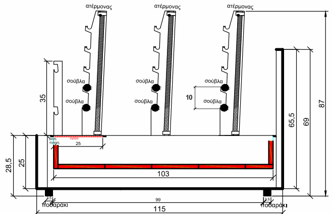
ΠΛΑΪΝΗ ΟΨΗ 3 ΑΞΙΟΝΑΣ
